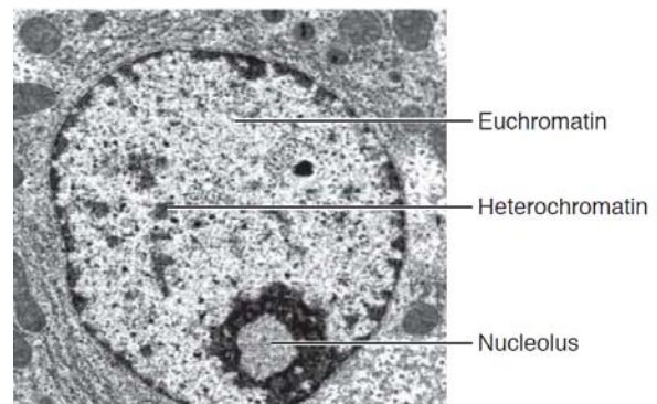
Nhân ở kỳ trung gian
