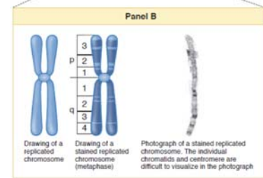
Panel B: NST eukaryote đã nhân đôi
