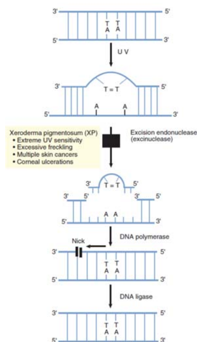
Sự hình thành dimer thymine và sửa chữa cắt
